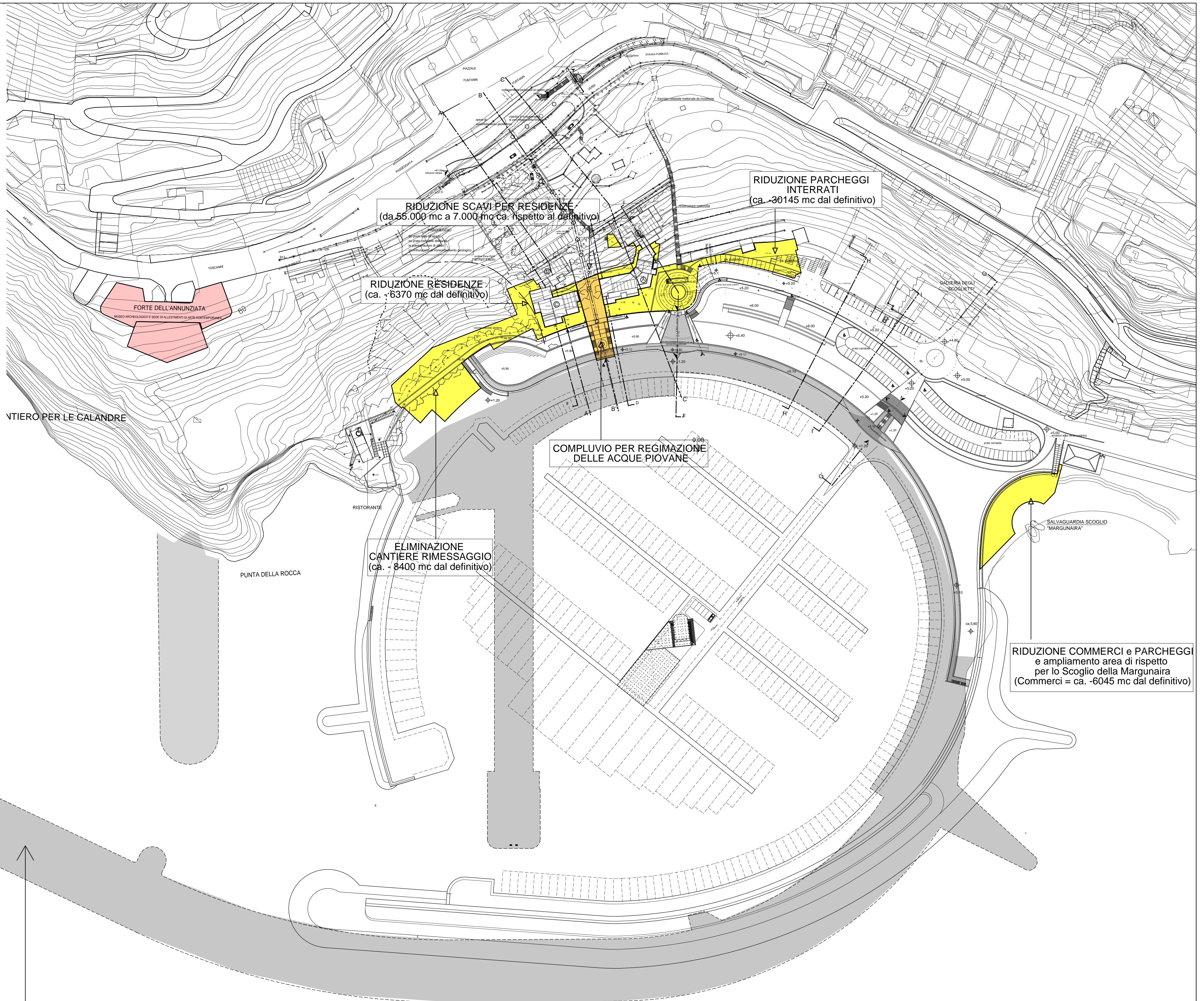
INGOMBRO DIGA PROGETTO DEFINITIVO (Luglio 2005)
